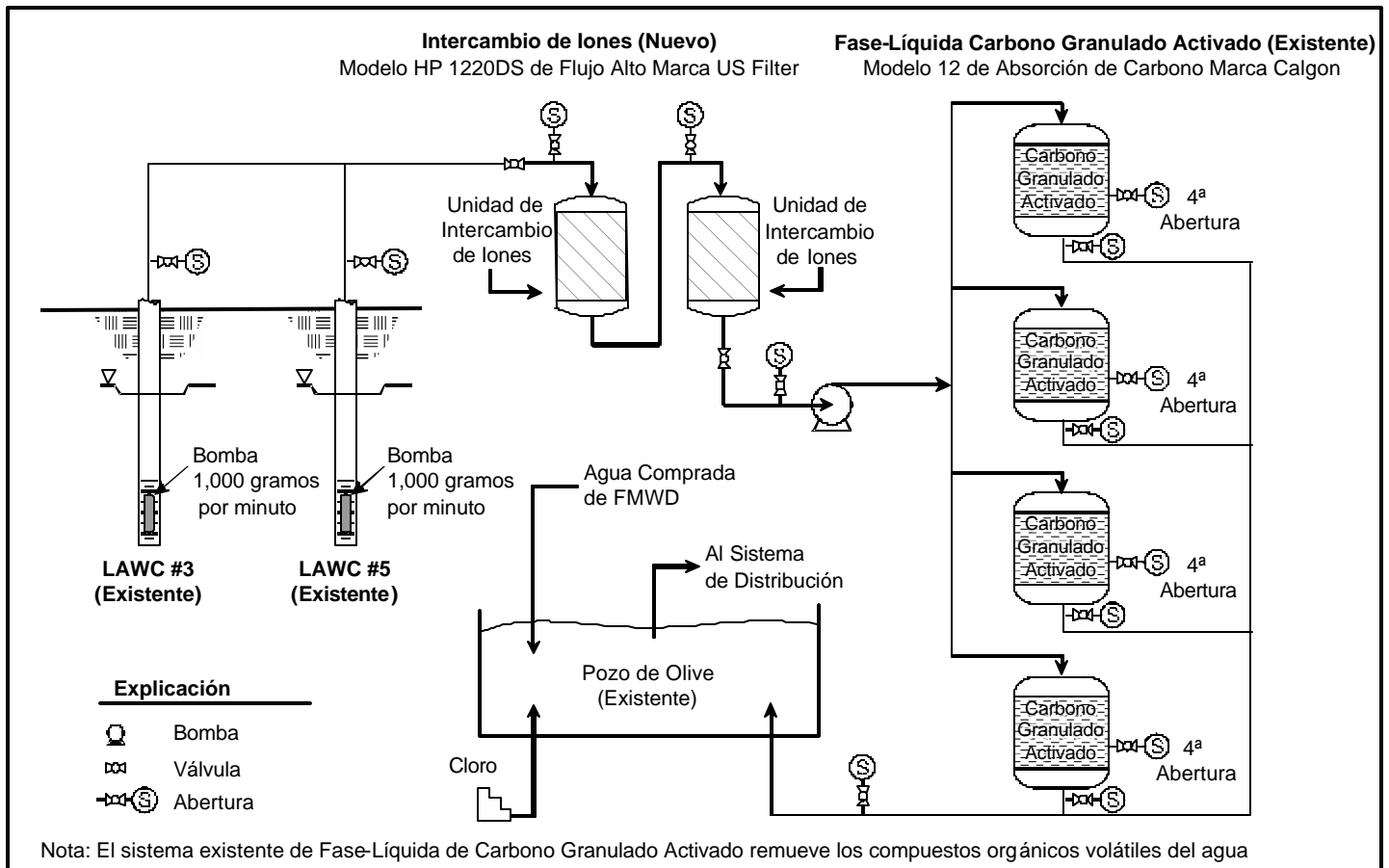
Dibujo 2. Diagrama del Proceso de Tratamiento del Agua
