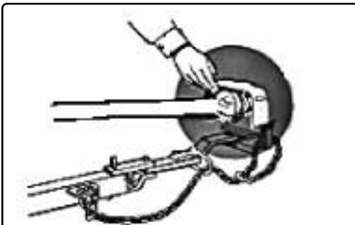
Accidentes de agarrado o atrapado pueden ocurrir entre el PTO y el protector, como es mostrado aquí.
